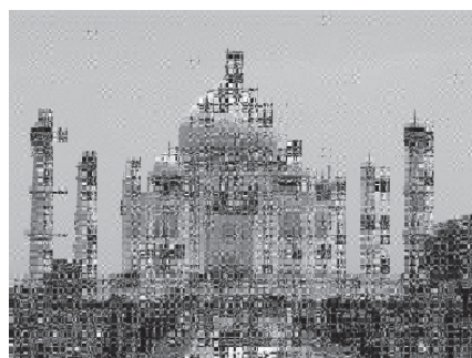
(d) Approximation 24 ( I_{24} ).
