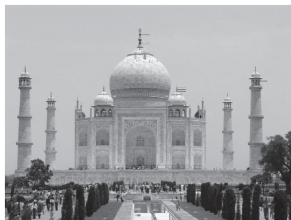
(h) Approximation 31 ( I_{31} ).
