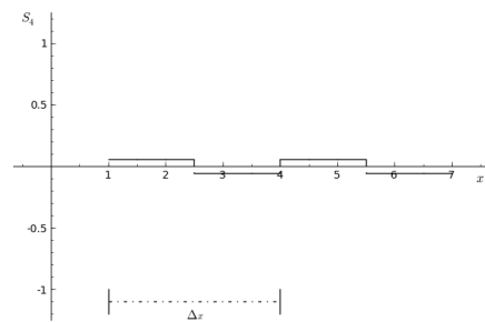
(d) S_4(x) .
