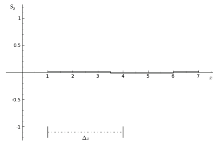
(b) S_2(x) .
