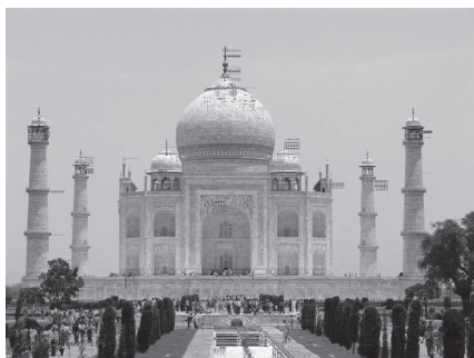
(g) Approximation 30 ( I_{30} ).
